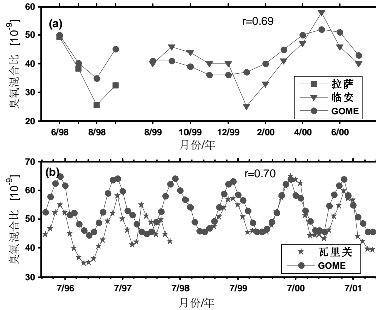
图4 GOME近地面层臭氧浓度（实心圆）同拉萨（实心方框），临安（下三角形），瓦里关山（星形）地面观测臭氧浓度的对比， r 为相关系数
