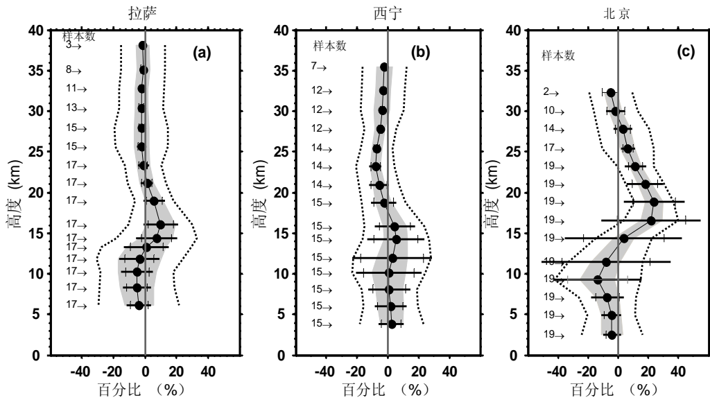
图1 GOME同3个站点臭氧探空对比，各层臭氧总量的相对偏差 \langle \text{GOME} - \text{sonde} \rangle / \langle \text{sonde} \rangle (圆点线)，标准偏差 (黑细线)，3倍标准误差 (误差棒)，相对的合成的随机误差 (灰影区)，合成的误差 (虚线)，带箭头数字表示该层样本数
