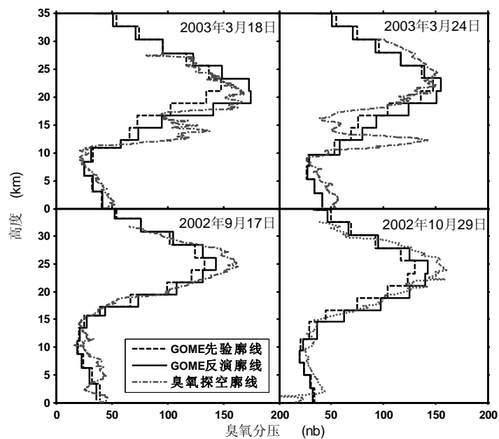
图 2 2002年秋季,2003年春季GOME臭氧资料先验廓线和反演廓线同北京臭氧探空对比
