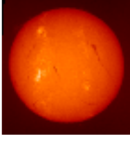
Sun
